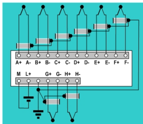
6ES7 231-7PF22-0XA0
