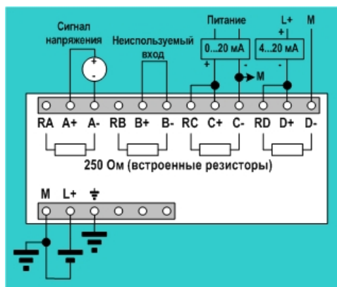
6ES7 231-0HC22-0XA0
